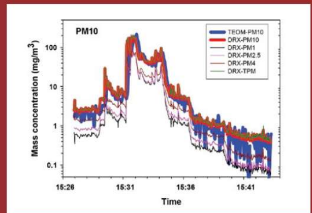
Vergleich der Massenkonzentration von Arizona Road Dust (A1) mittels Messung durch das DustTrak DRX und das TEOM mit PM10 Einlasskonditionierer.
