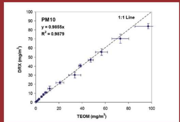
Lineare Übereinstimmung zwischen DustTrak DRX und TEOM für die Messung der Massenkonzentration von Arizona Road Dust (A1). Das TEOM lief mit einem PM10 Einlasskonditionierer.
