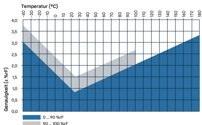
Genauigkeit der HMP4 Feuchtemessung in Abhängigkeit von der Temperatur
