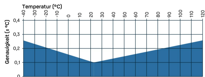
Genauigkeit der HMP3 Temperaturmessung über den gesamten Messbereich
